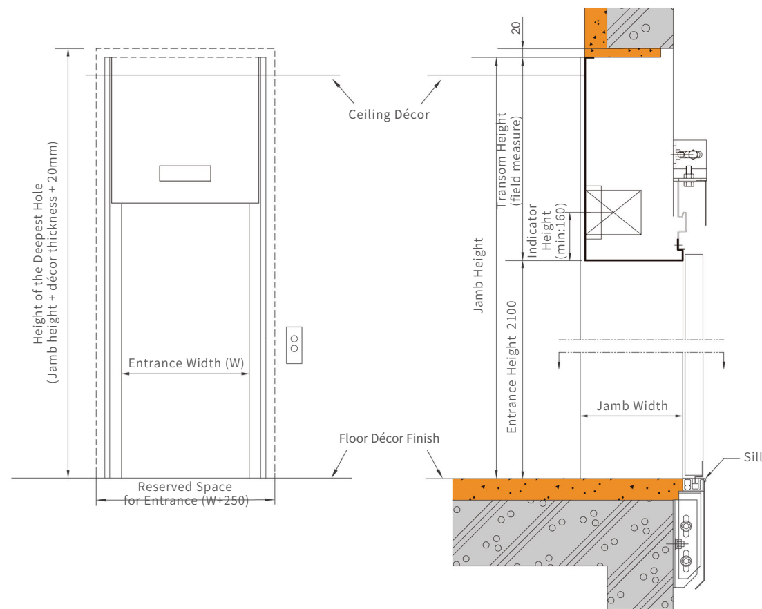
A-A Section
