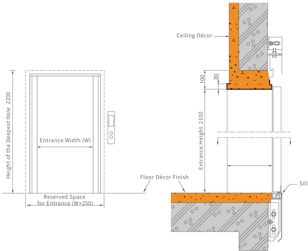
A-A Section
