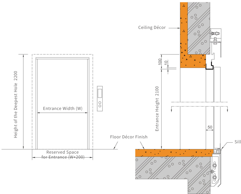
A-A Section
